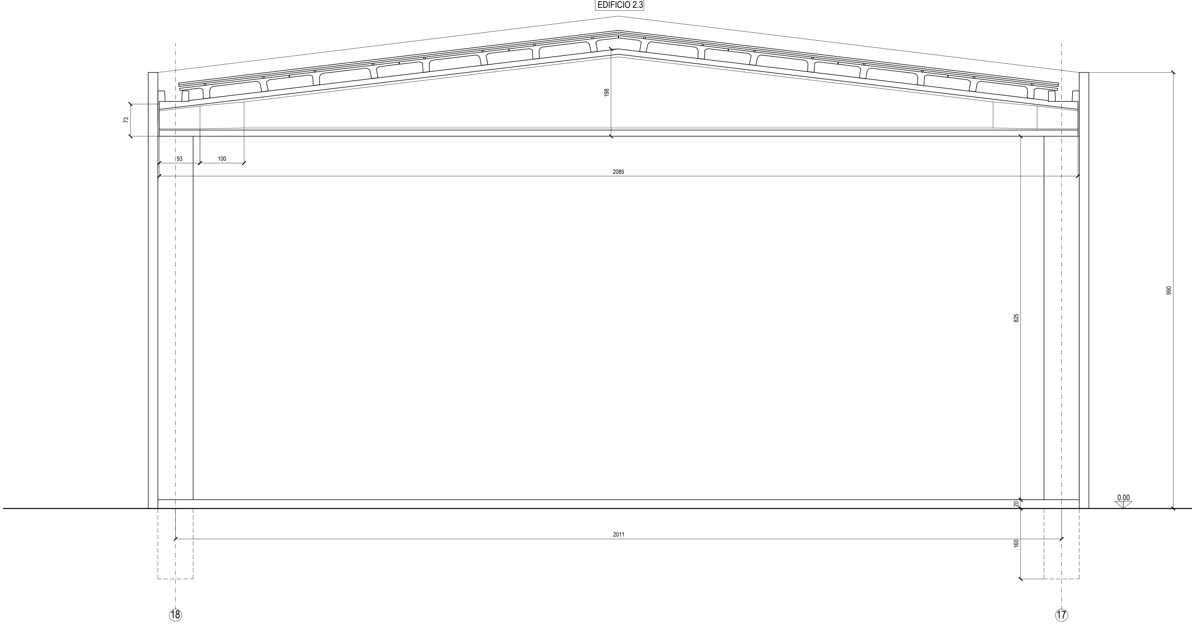
PROSPETTO D3 SCALA 1:100
