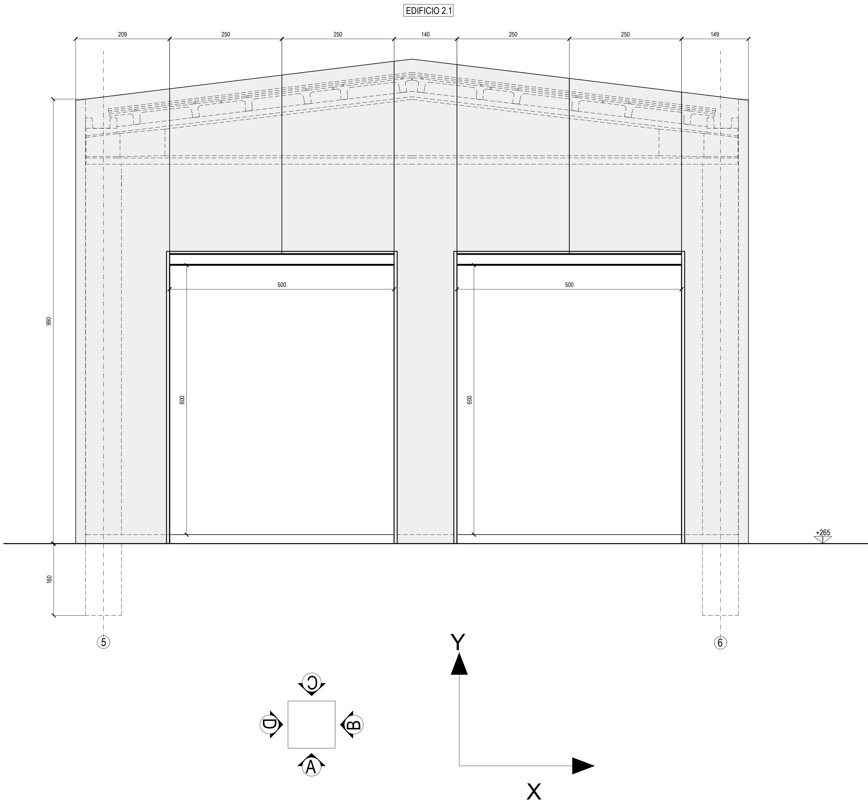
PROSPETTO B3 SCALA 1:100
