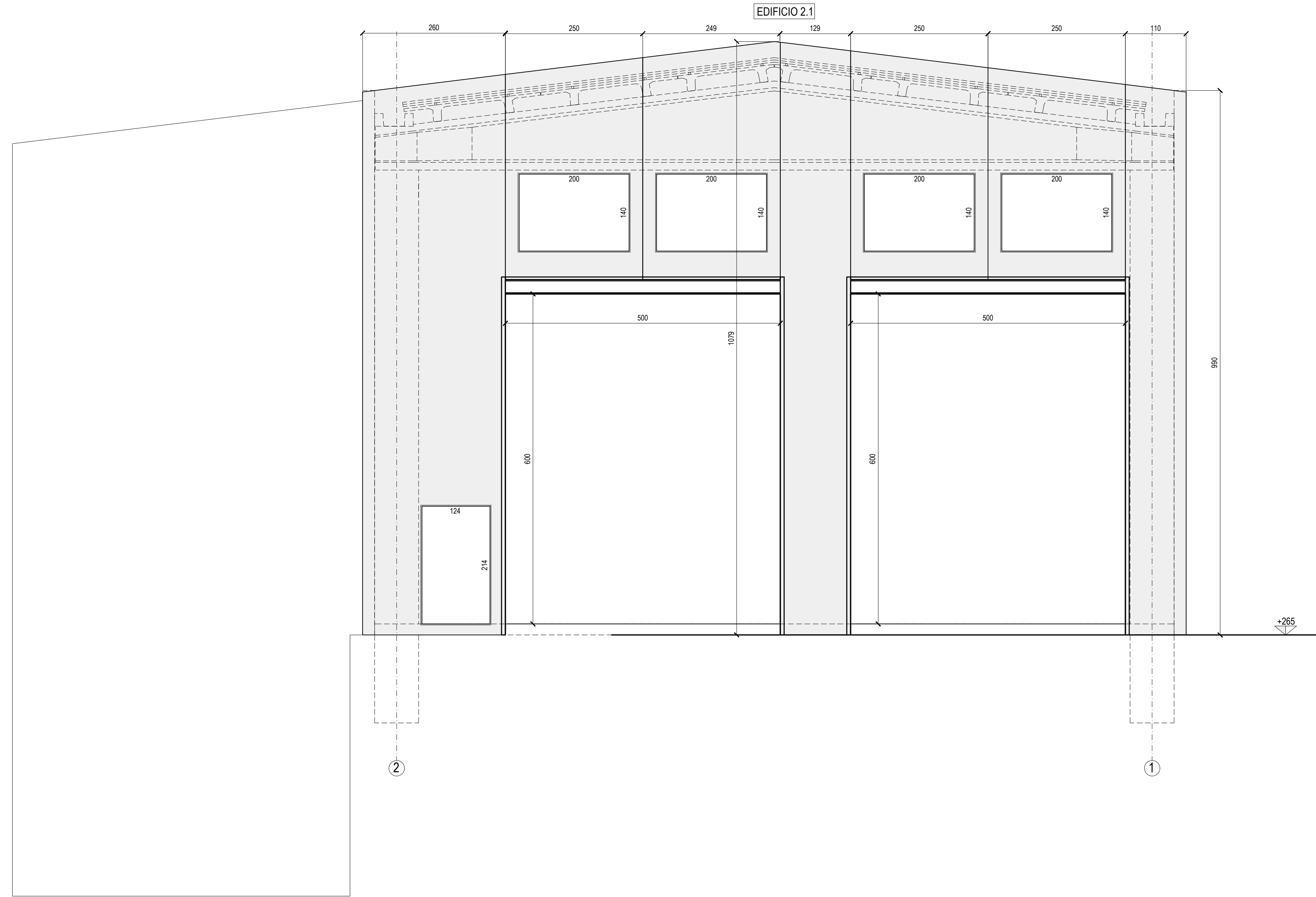
PROSPETTO D1 SCALA 1:100
