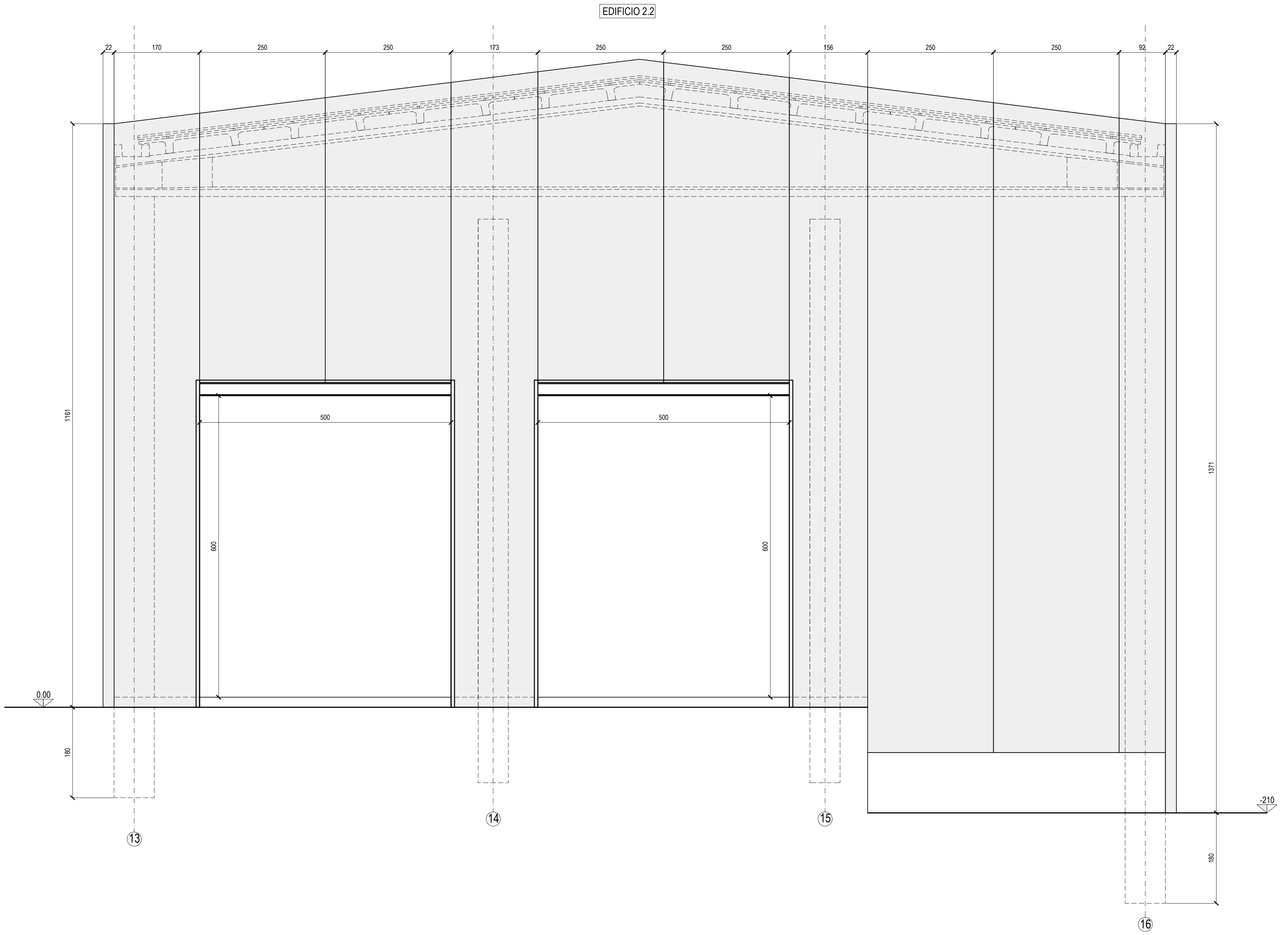
PROSPETTO B2 SCALA 1:100
