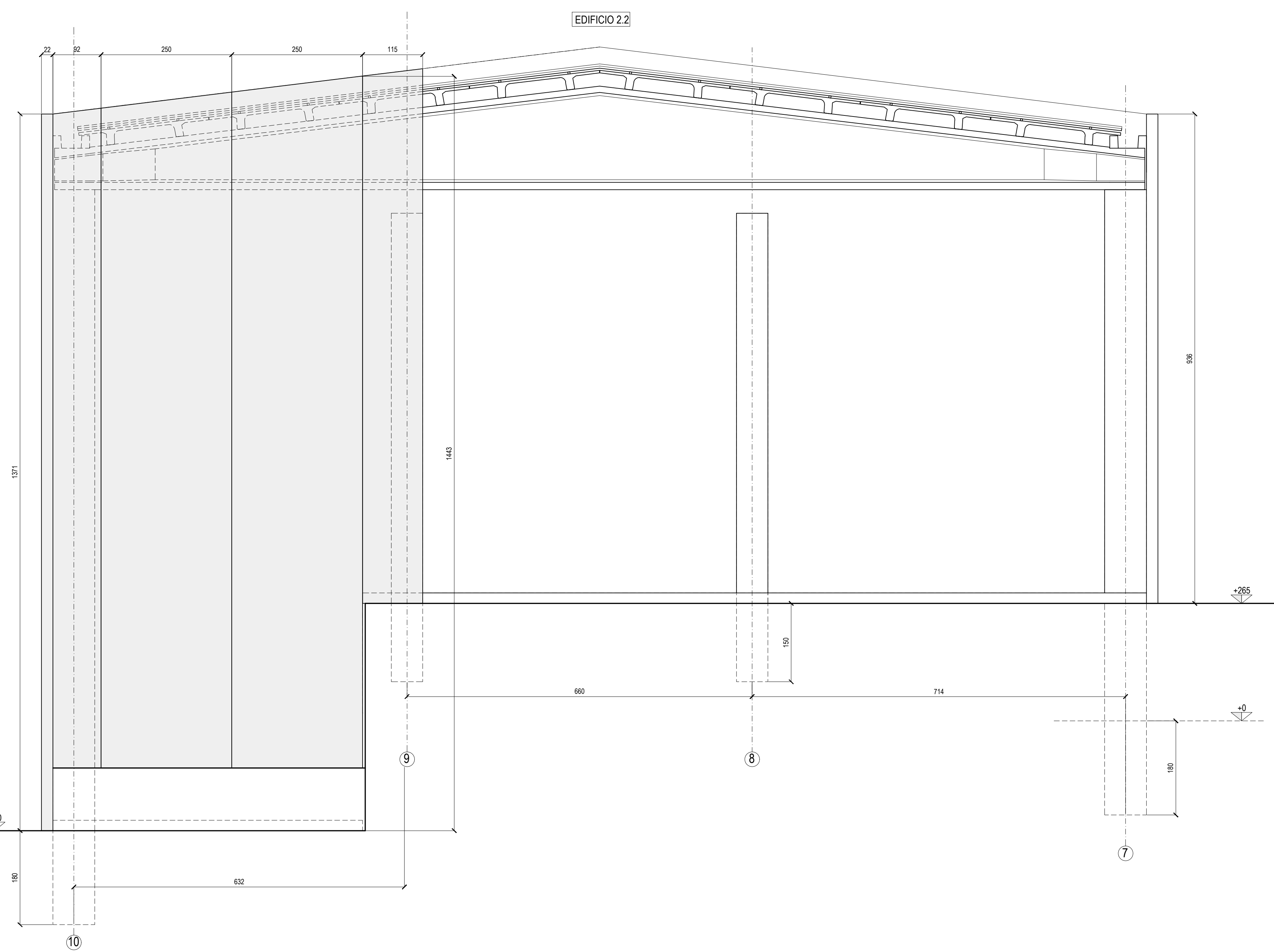
PROSPETTO D2 SCALA 1:100
