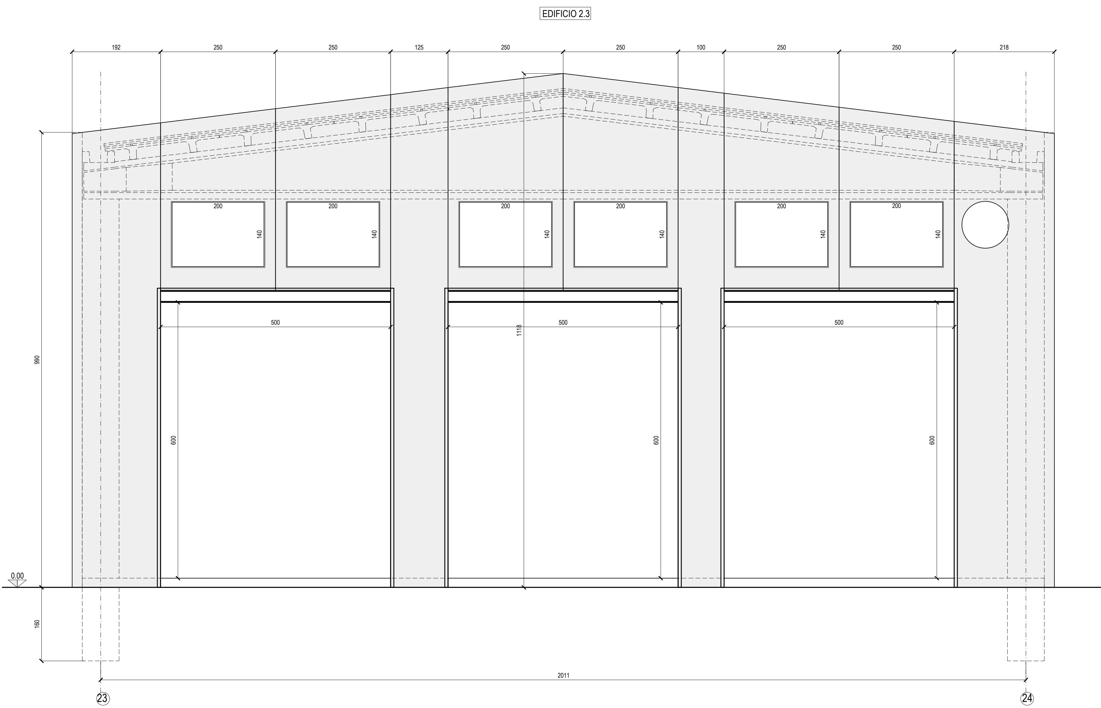
PROSPETTO B1 SCALA 1:100
