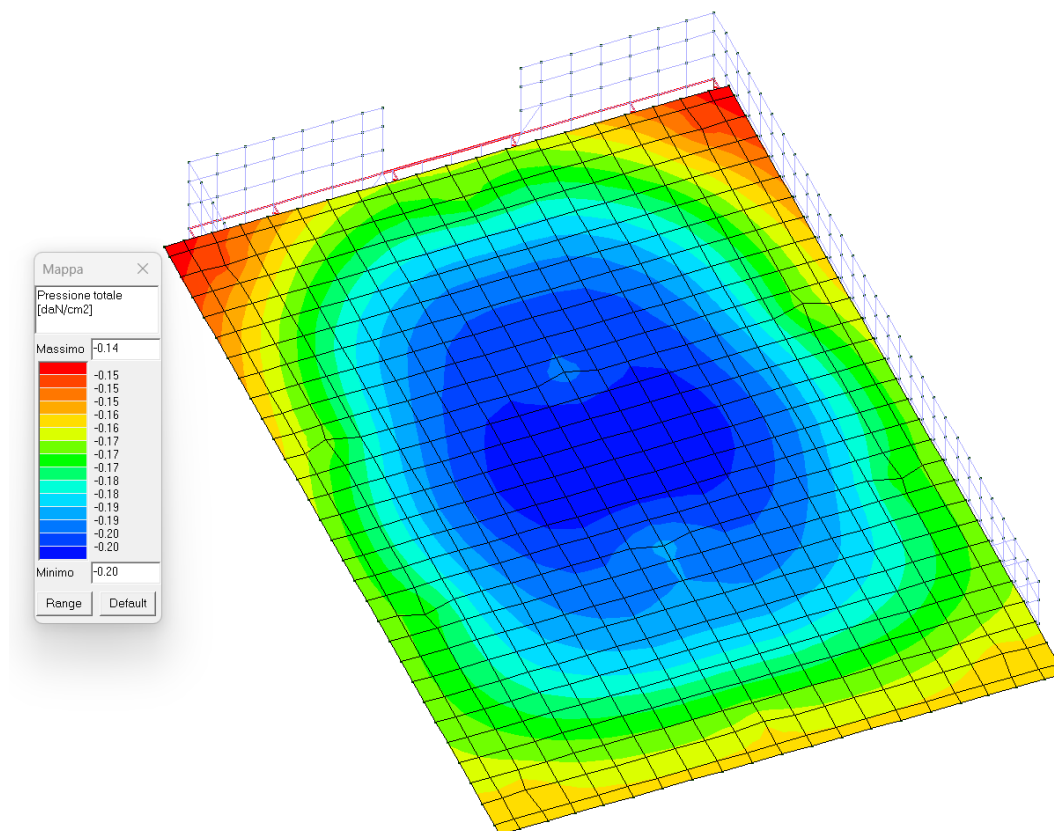
Figura 20 - Pressione totale per la combinazione 164) SLE (perm.)
