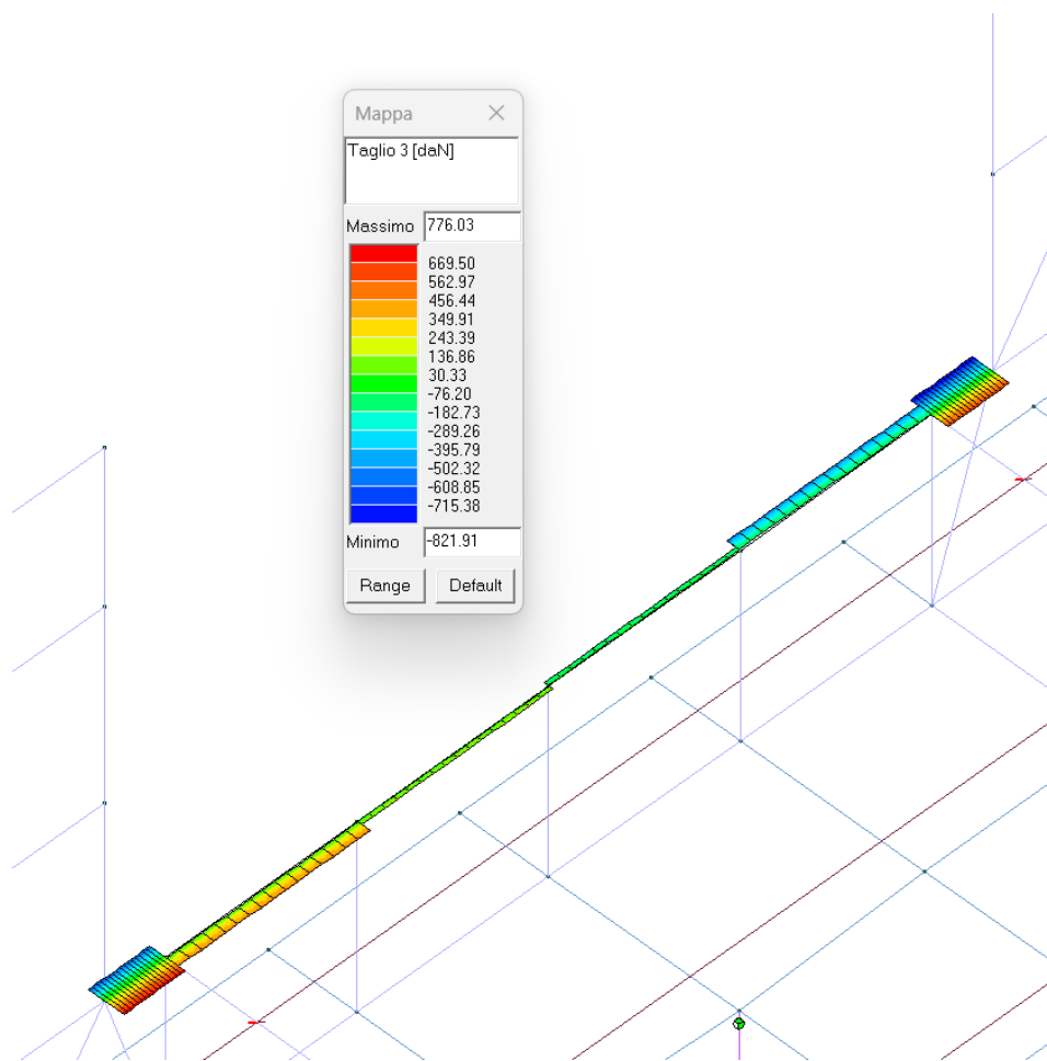
Figura 35 - SFORZO DI TAGLIO T3 SULLA TRAVE
