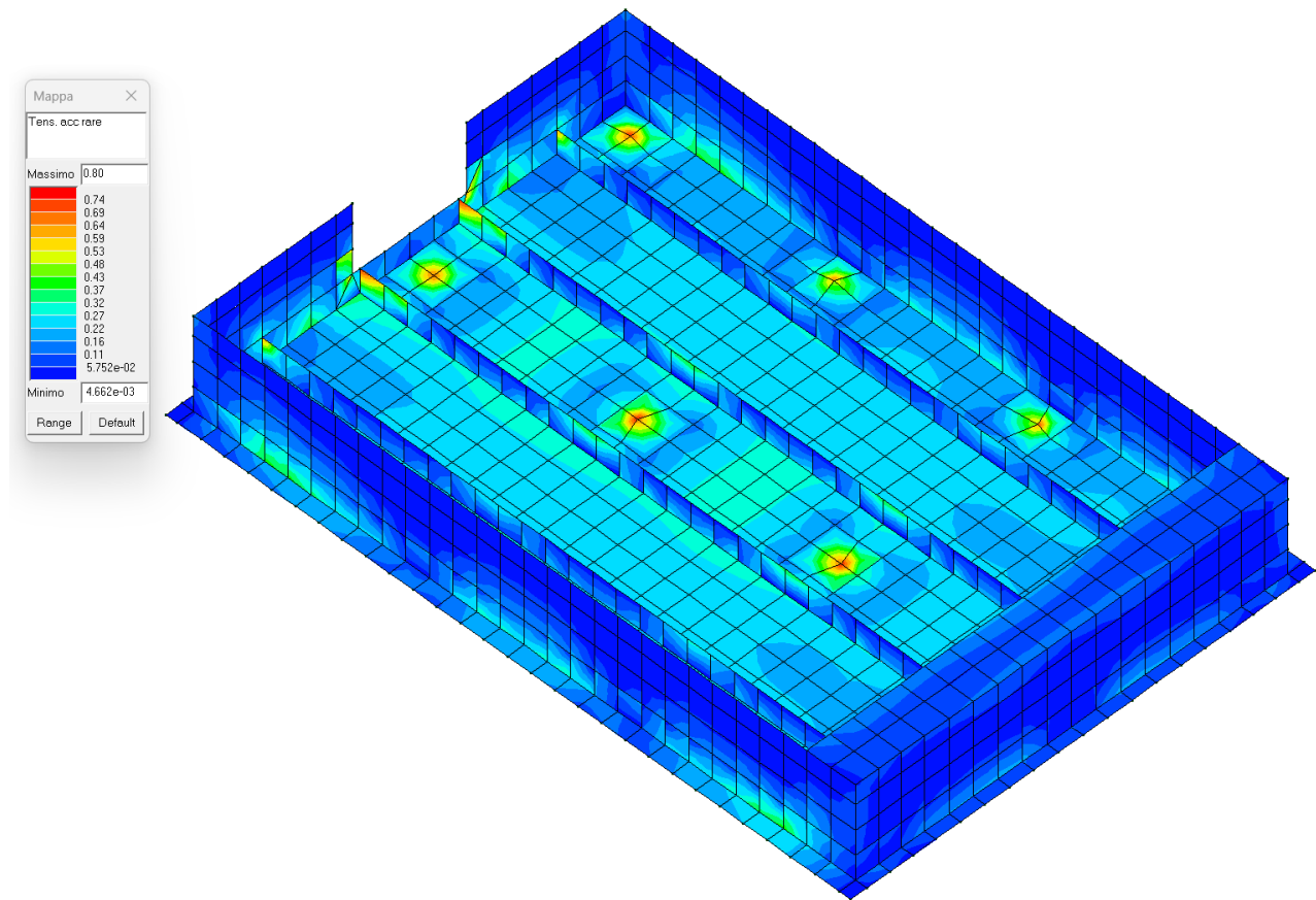
Figura 46 - SLE tens. acciaio Comb. Rare: valore minore o uguale a 1 per verifica positiva
