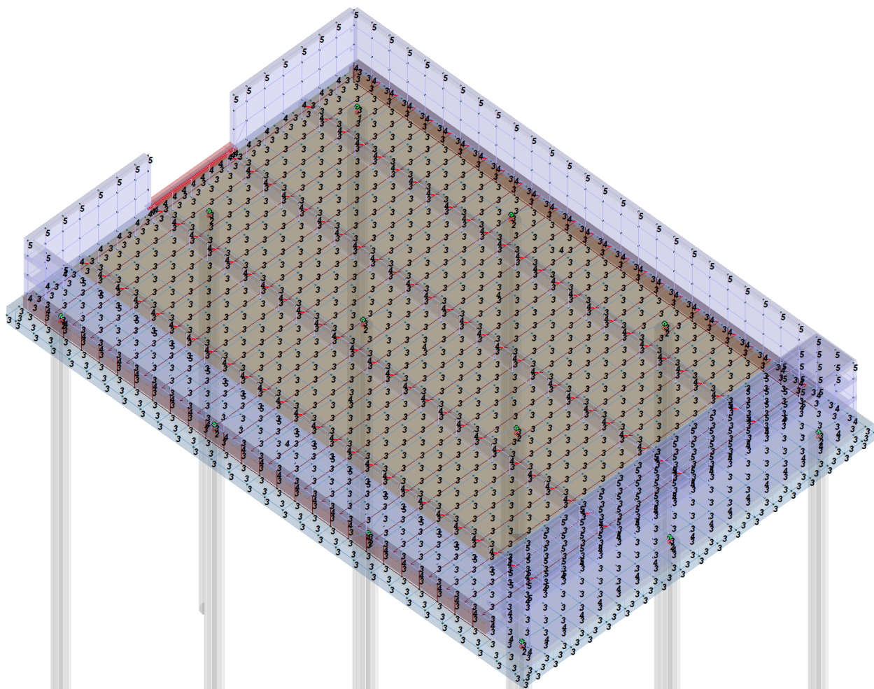
Figura 7 - Numerazione impalcati
