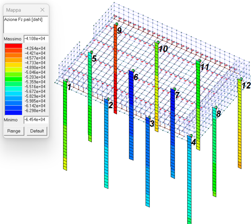
Figura 25- MAX Azione Fz pali [daN] per la combinazione 194) SLU (SLV sism.)
