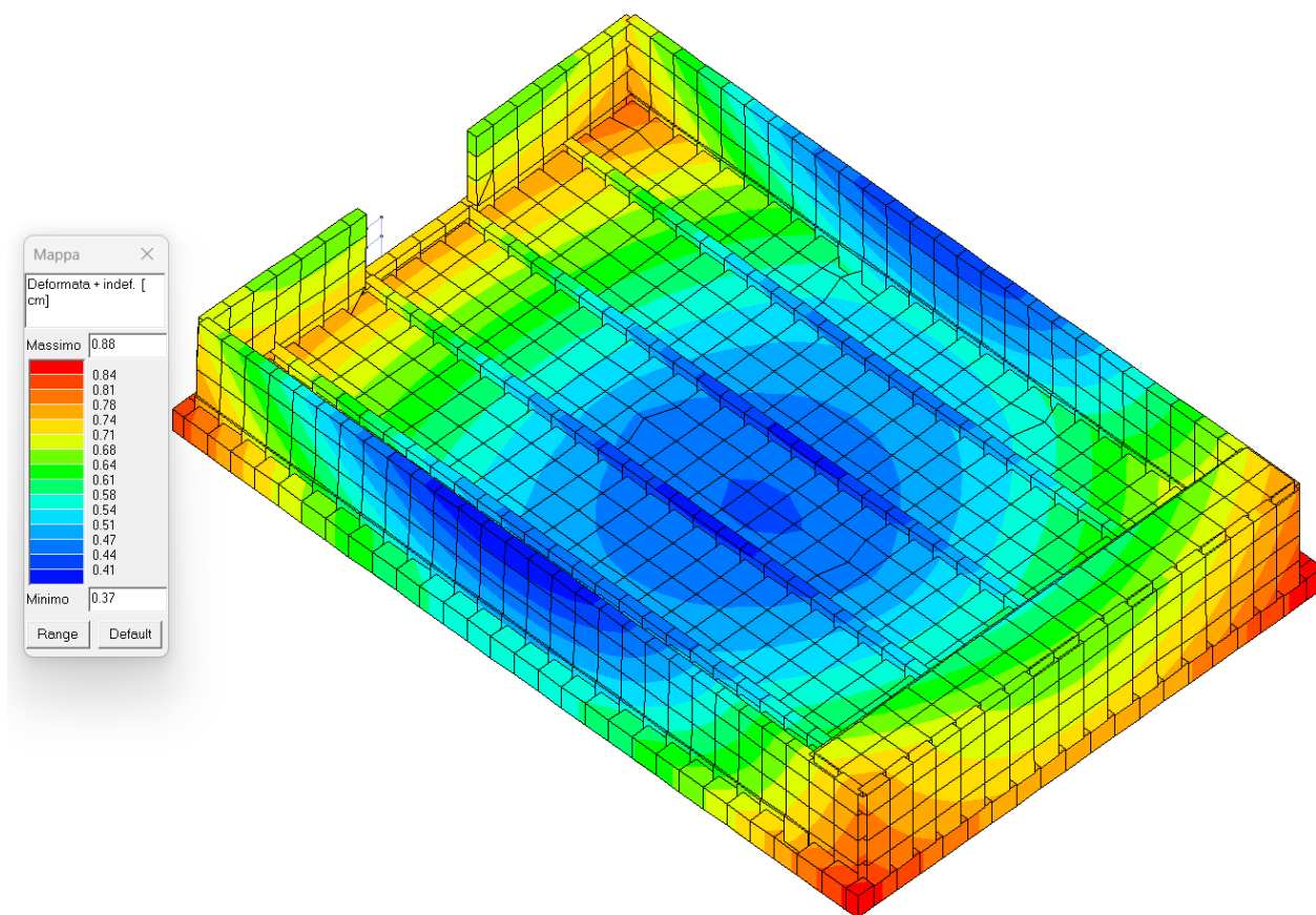
Figura 27 - MAX Deformata per la combinazione 79) SLU A1
