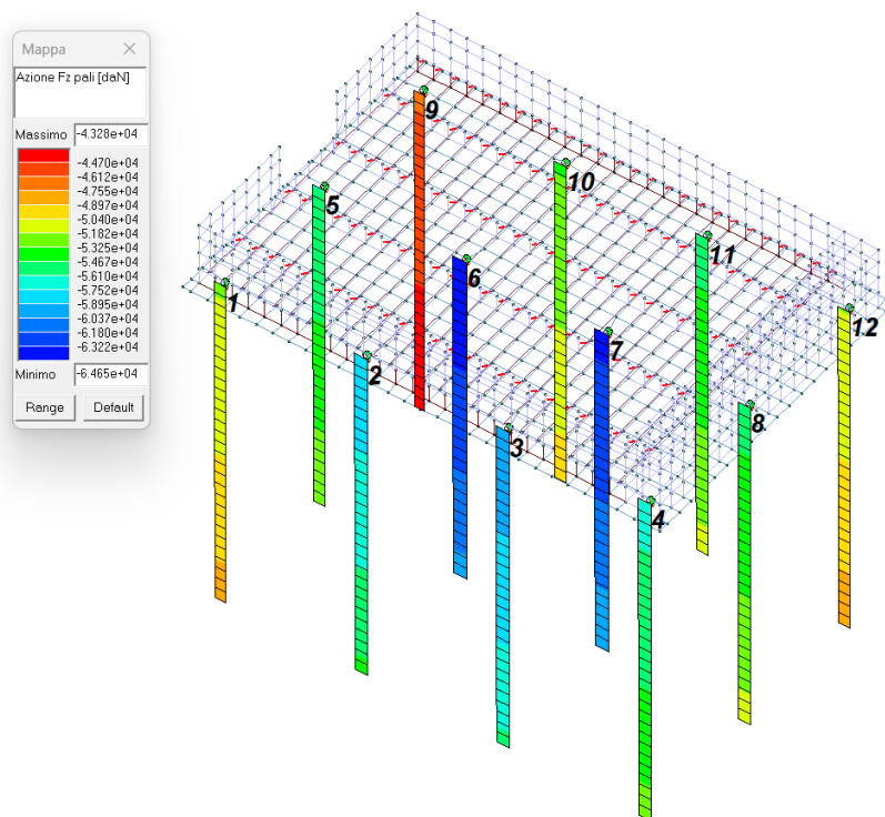
Figura 26 - MAX Azione Fz pali [daN] per la combinazione 226) SLE (SLD Danno sism.)
