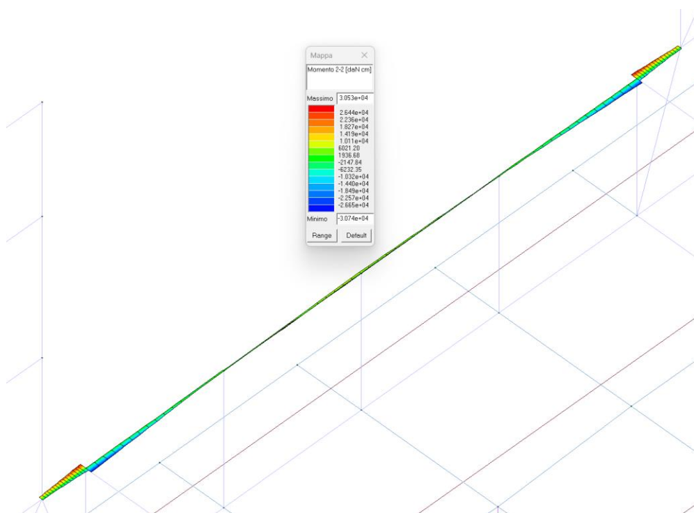
Figura 36 - MOMENTO M 2-2 SULLA TRAVE
