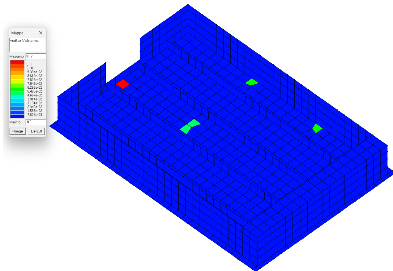
Figura 44 – SLU Verifica a taglio nella direzione principale lato calcestruzzo: valore minore o uguale a 1 per verifica positiva
