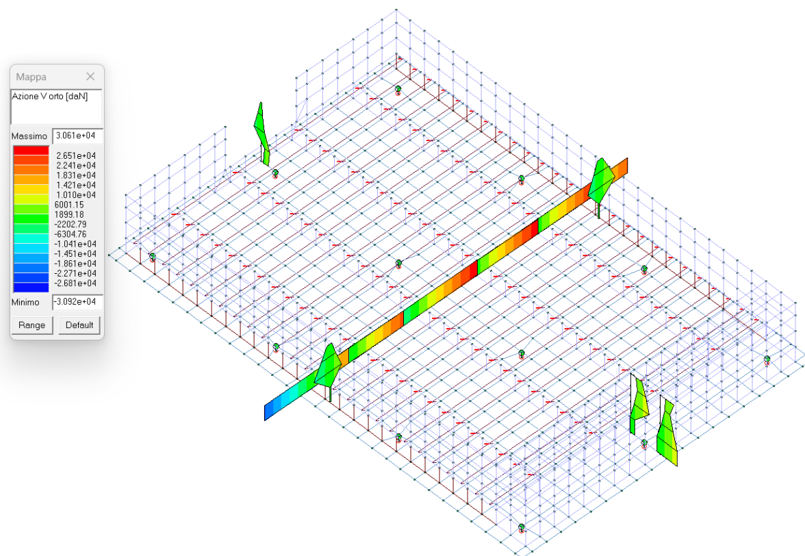
Figura 40 - AZIONE V ORTO. Tale azione è quella complessiva agente sul macroelemento.
