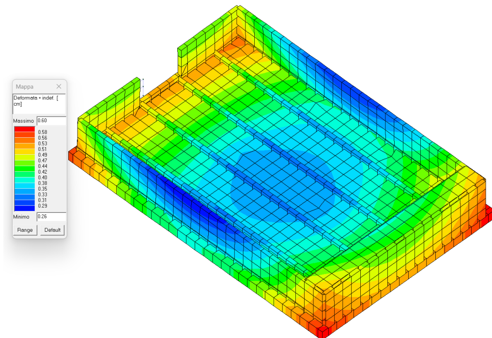
Figura 28 - MAX Deformata per la combinazione 144) SLE (rara)
