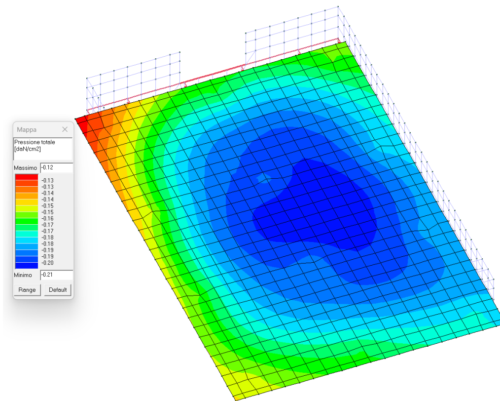
Figura 18 - MAX Pressione totale per la combinazione 189) SLU A1 (SLV sism.)
