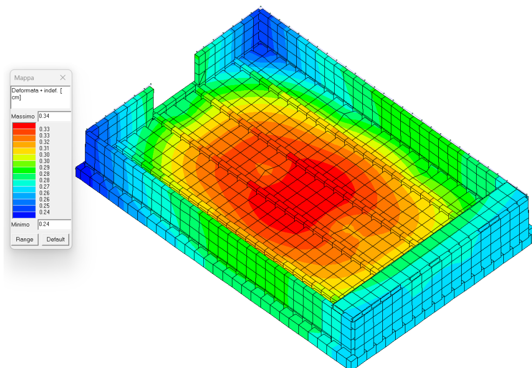
Figura 30 - MAX Deformata per la combinazione 164) SLE (perm.)
