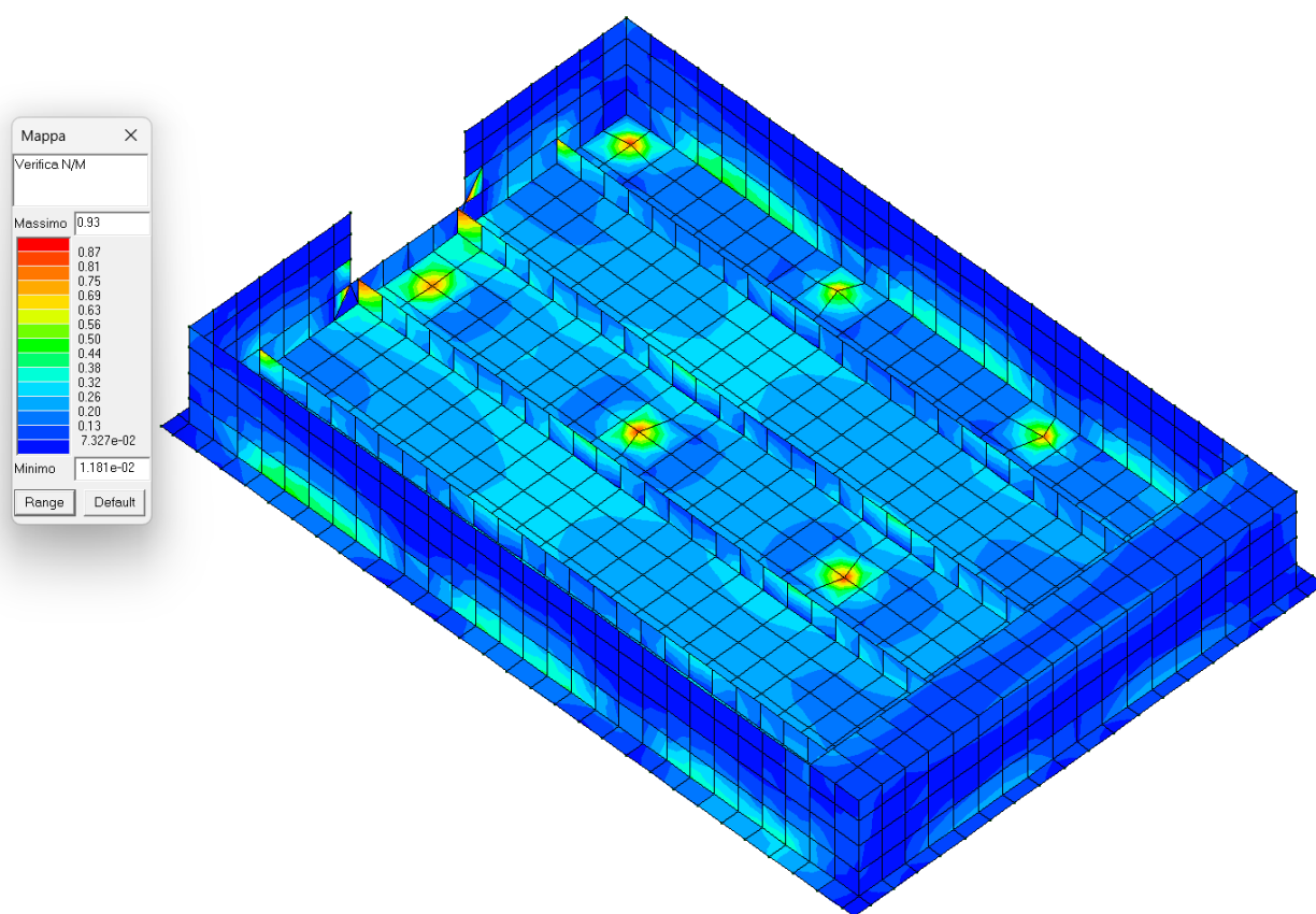
Figura 43 - SLU Verifica a pressoflessione rapporto E_d/R_d : valore minore o uguale a 1 per verifica positiva
