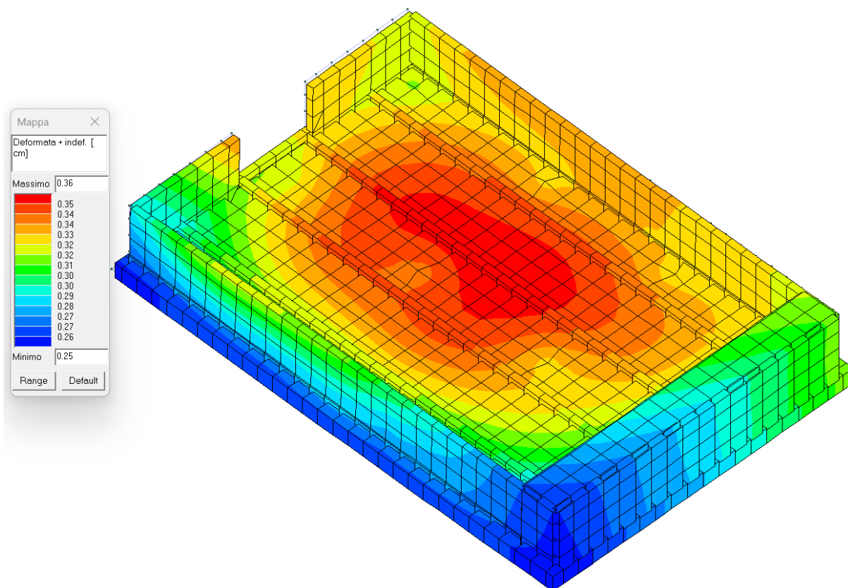
Figura 31 - MAX Deformata per la combinazione 193) SLU A1 (SLV sism.)
