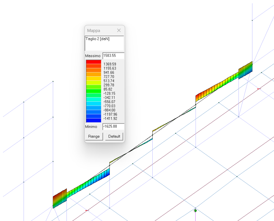
Figura 34 - SFORZO DI TAGLIO T2 SULLA TRAVE
