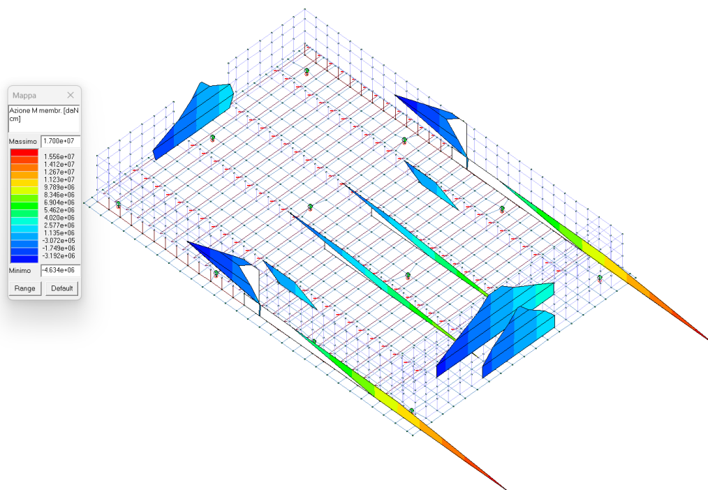
Figura 41 - AZIONE M MEMBR. Tale azione è quella complessiva agente sul macroelemento.
