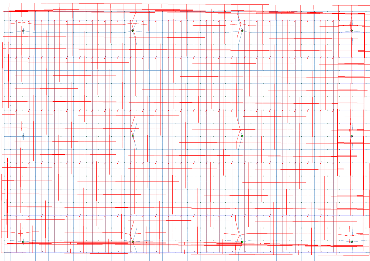
Figura 13 - II° periodo proprio (Prevalentemente traslazione lungo l'asse y)
