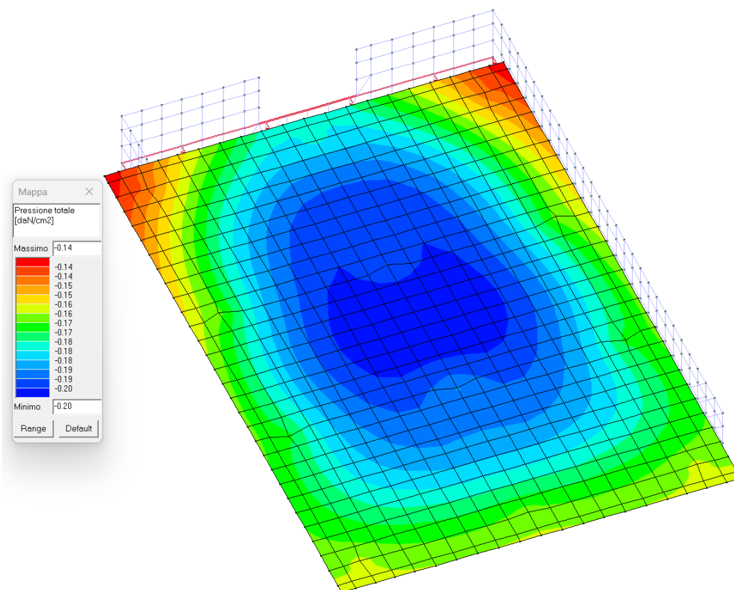
Figura 16 - MAX Pressione totale per la combinazione 155) SLE(rara)
