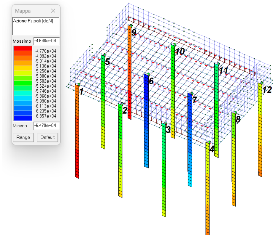
Figura 24 - MAX Azione Fz pali [daN] per la combinazione 164) SLE (perm.)
