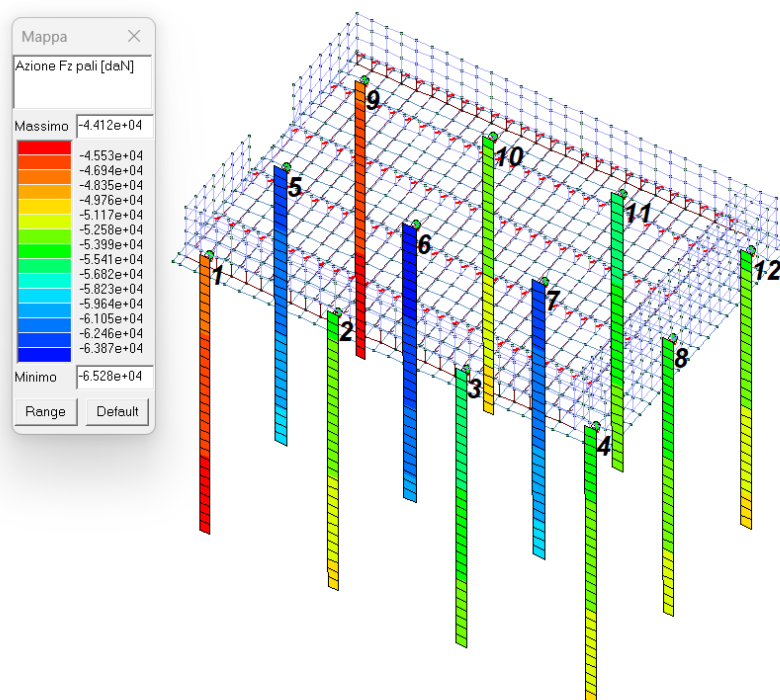
Figura 23 - MAX Azione Fz pali [daN] per la combinazione 155) SLE(rara)
