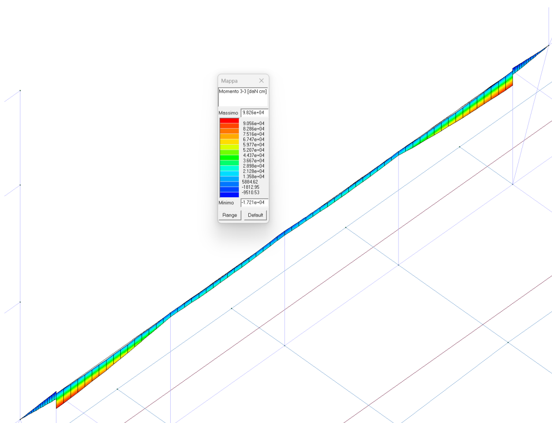
Figura 37 - MOMENTO M3-3 SULLA TRAVE
