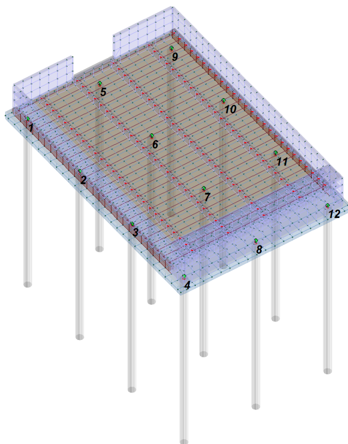
Figura 4 - Numerazione Pali di Fondazione
