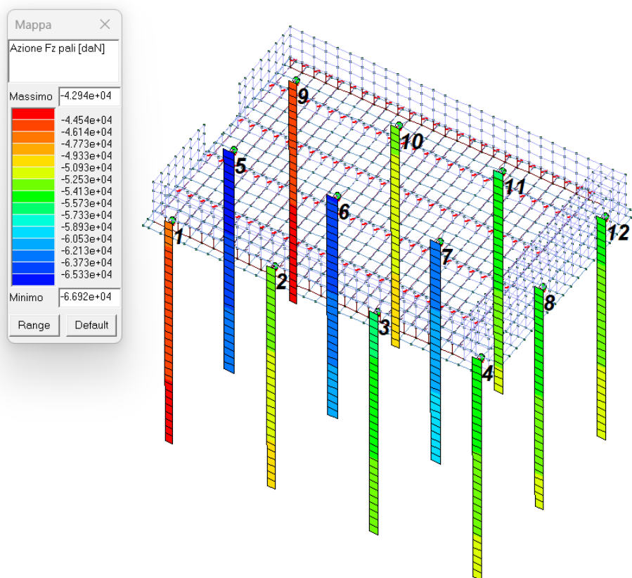
Figura 21 - MAX Azione Fz pali [daN] per la combinazione 102) SLU A1
