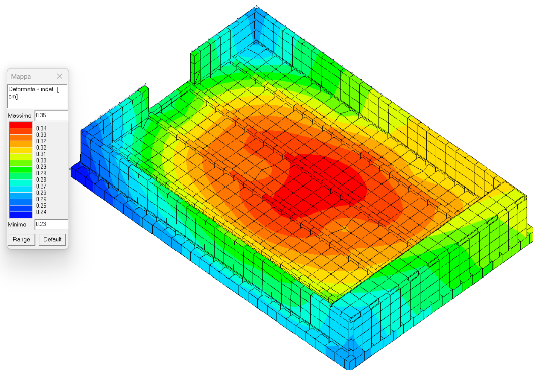
Figura 32 - MAX Deformata per la combinazione 219) SLE (SLD danno sism.)
