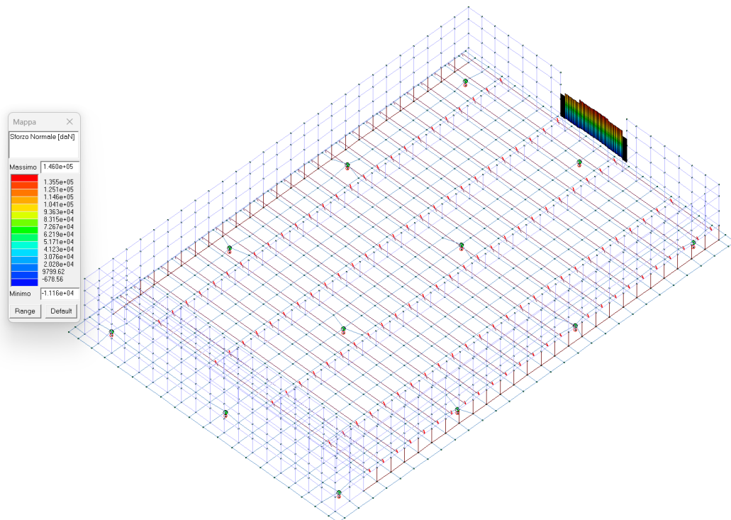
Figura 33 - SFORZO NORMALE N SULLA TRAVE
