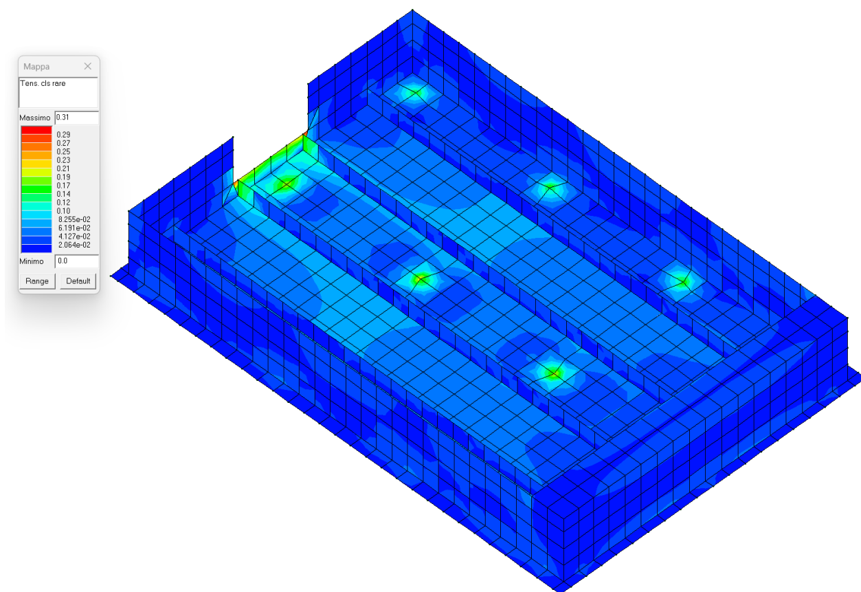
Figura 45 - SLE Tensione cls Comb. Rare: valore minore o uguale a 1 per verifica positiva
