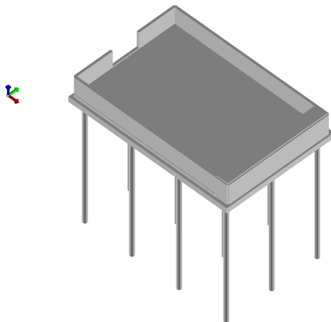
Figura 2 - Vista anteriore solida del modello
