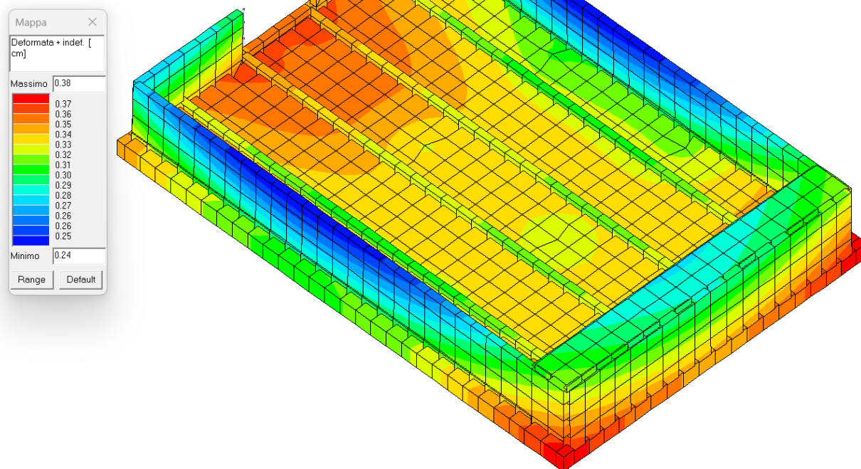
Figura 29 - MAX Deformata per la combinazione 159) SLE (freq)
