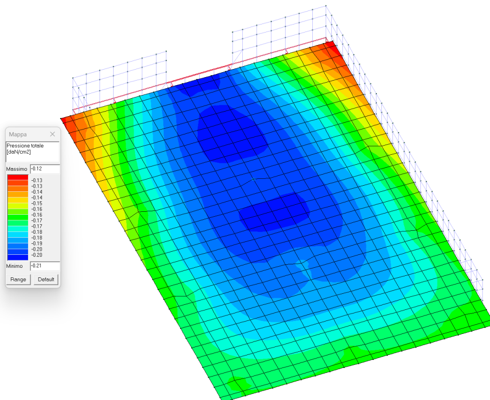
Figura 15 - MAX Pressione totale per la combinazione 102) SLU A1
