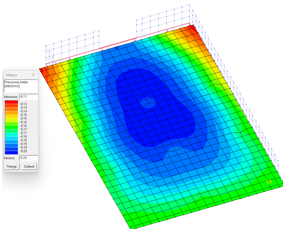
Figura 16 - MAX Pressione totale per la combinazione 155) SLE(rara)
