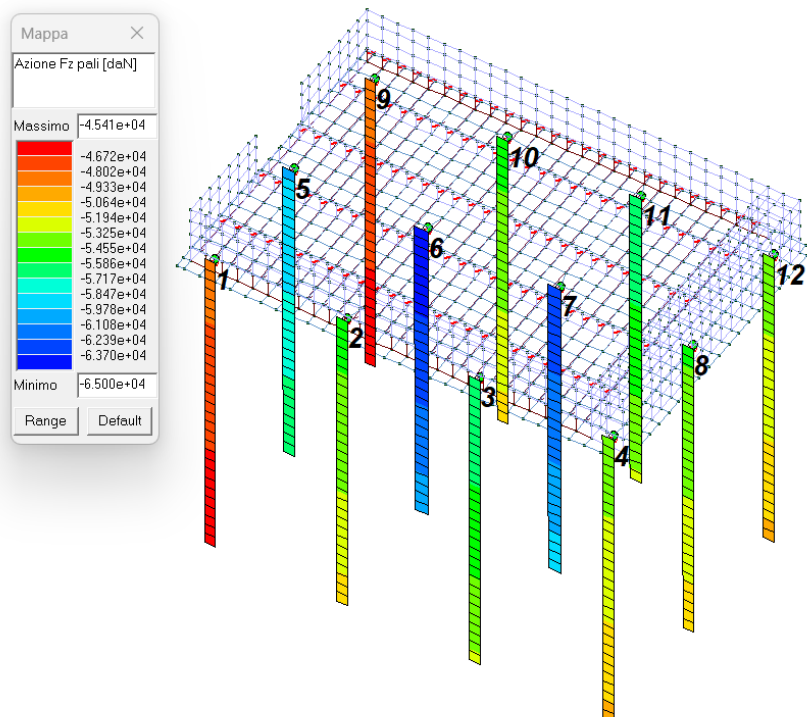
Figura 22 - MAX Azione Fz pali [daN] per la combinazione 159) SLE(freq.)
