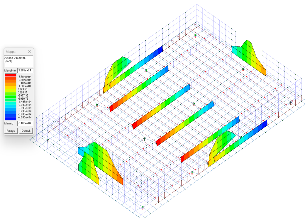
Figura 39- AZIONE V MEMBR. Tale azione è quella complessiva agente sul macroelemento.
