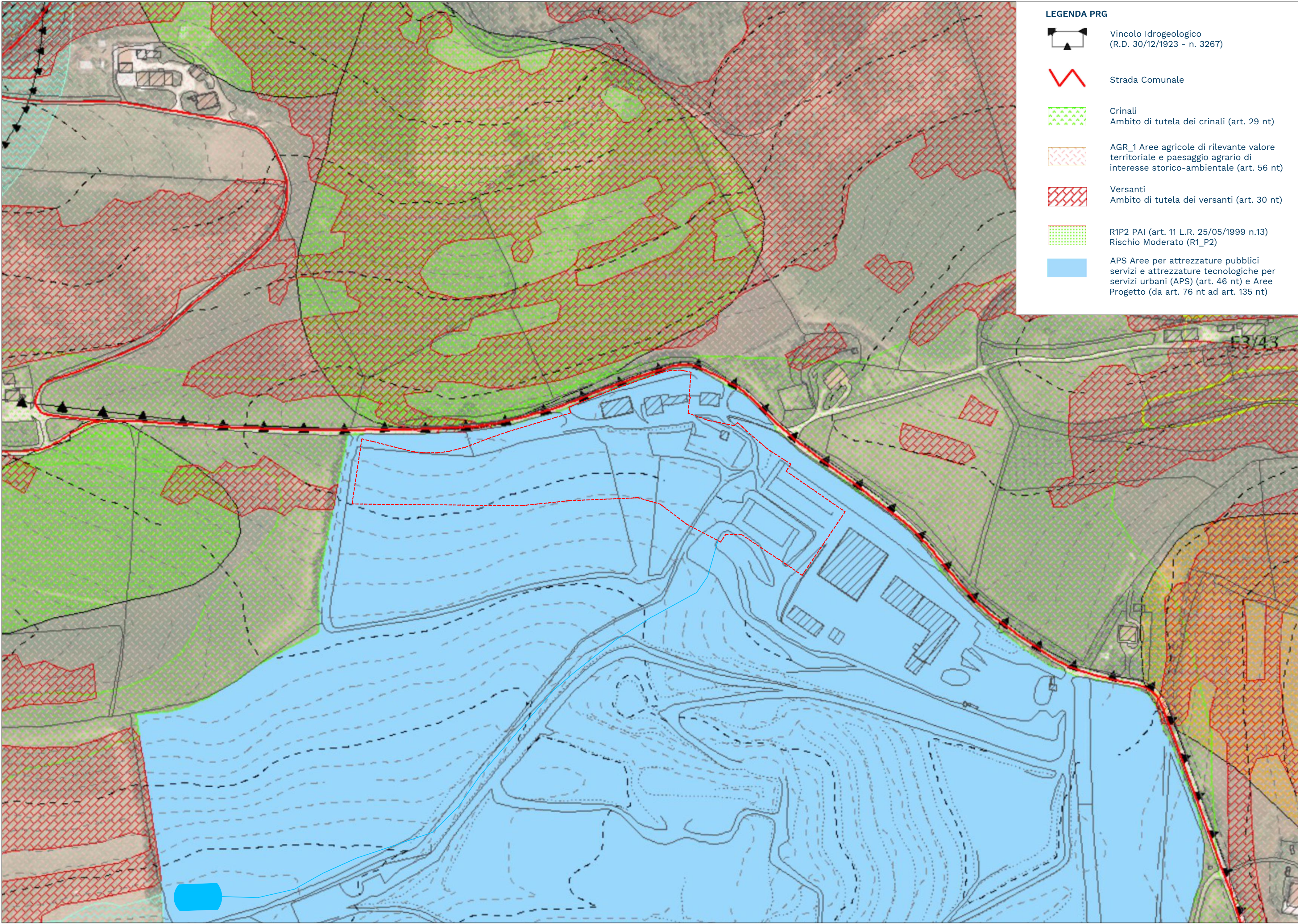
STRALCIO PRG CON SOVRAPPOSIZIONE LAYOUT DI PROGETTO - SCALA 1:2000
