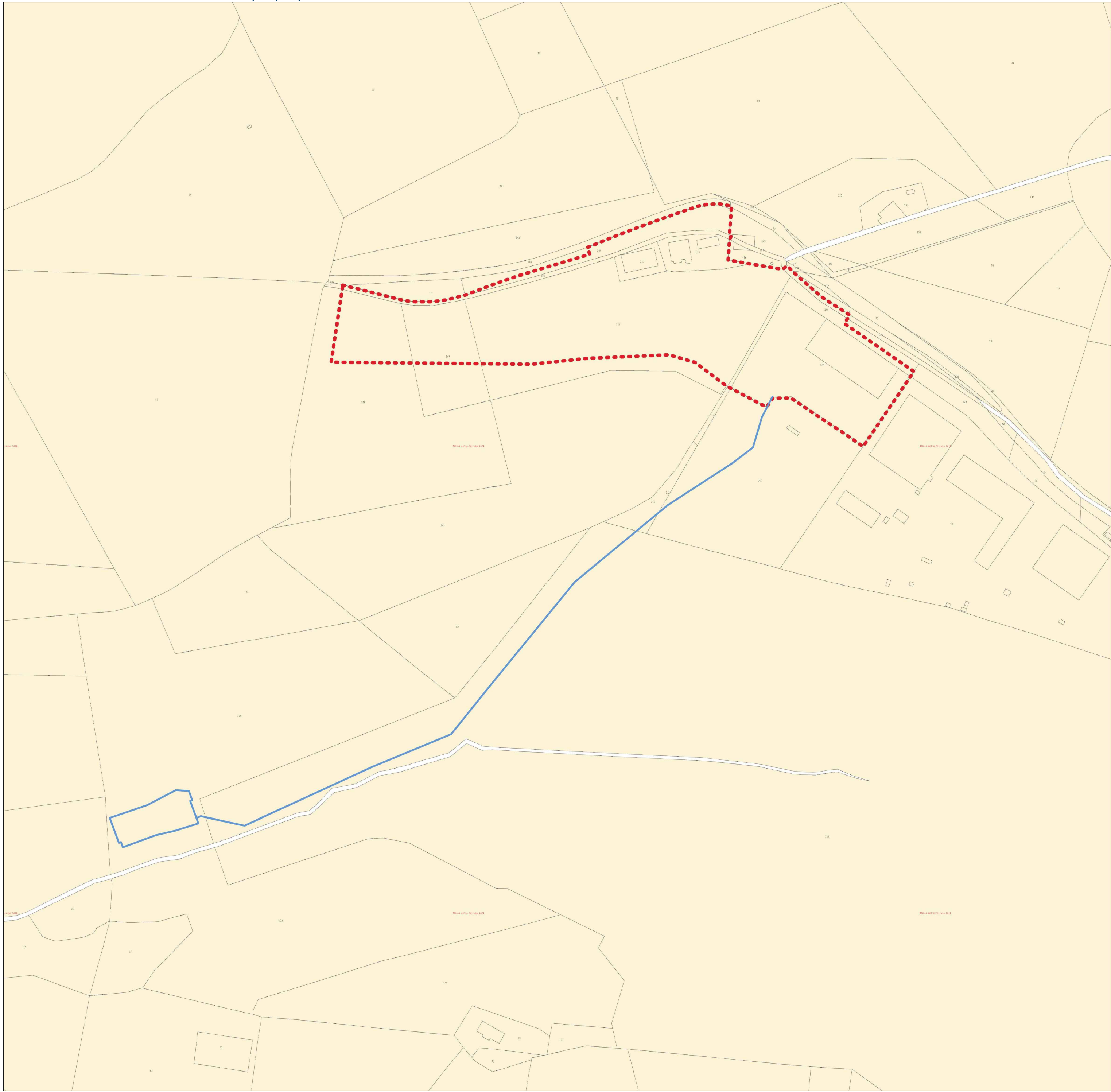
STRALCIO PLANIMETRIA CATASTALE - SCALA 1:2000 BIDIGESTORE: FOGLIO 111 - P.LLE 146, 147, 125, 142, 117, 119, 145, 131, 126 - FOGLIO 110 - P.LLE 144 BACINO DI LAMINAZIONE: FOGLIO 111 - P.LLE 148, 140, 132, 136
