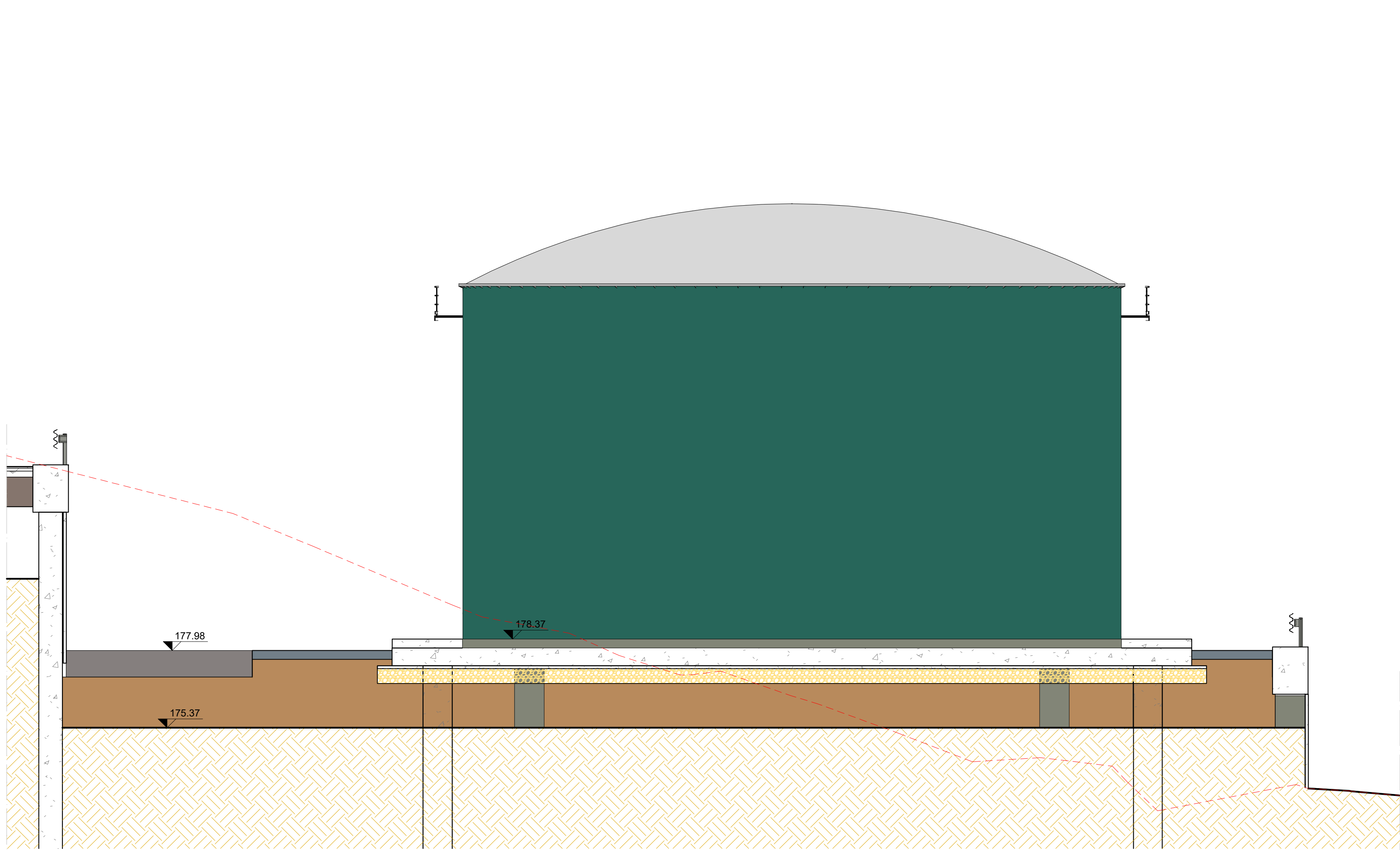
sezione B-B
