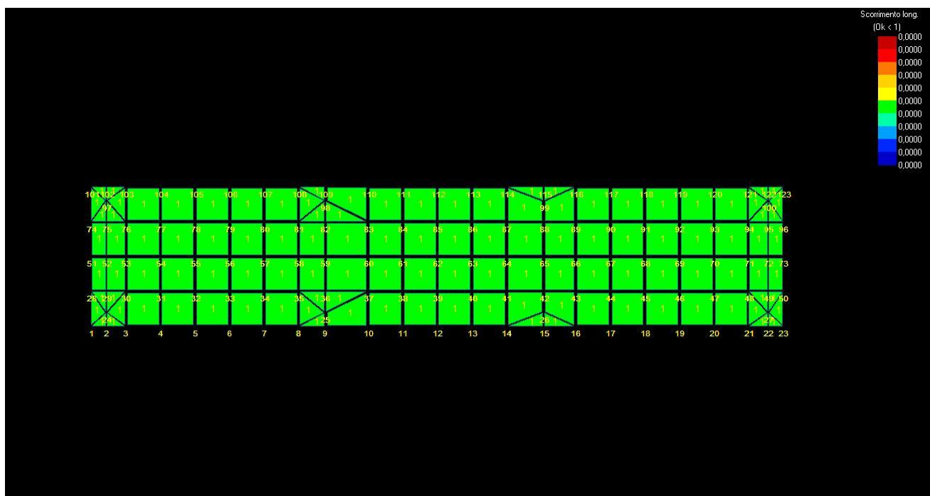
Figura 4 - verifica portanza longitudinale
