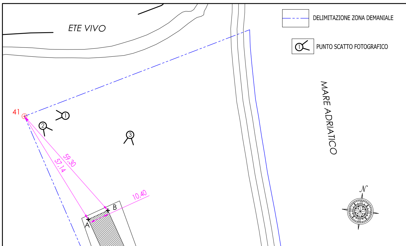
PARTICOLARE MONOGRAFIE
