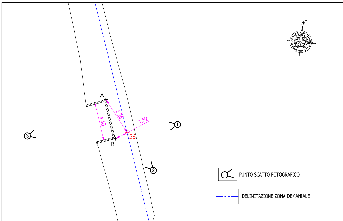
PARTICOLARE MONOGRAFIE
