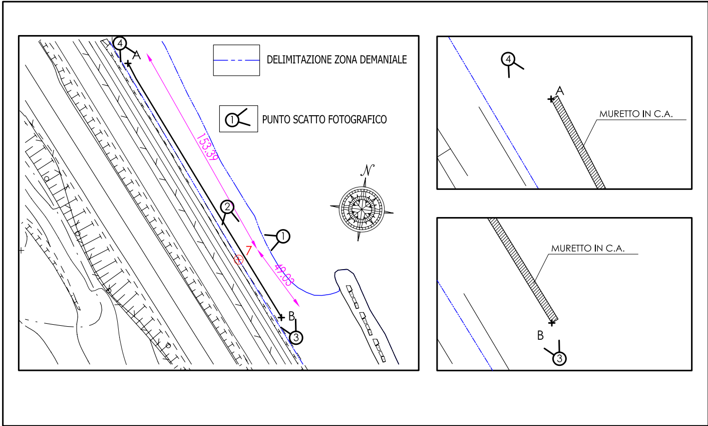
PARTICOLARE MONOGRAFIE
