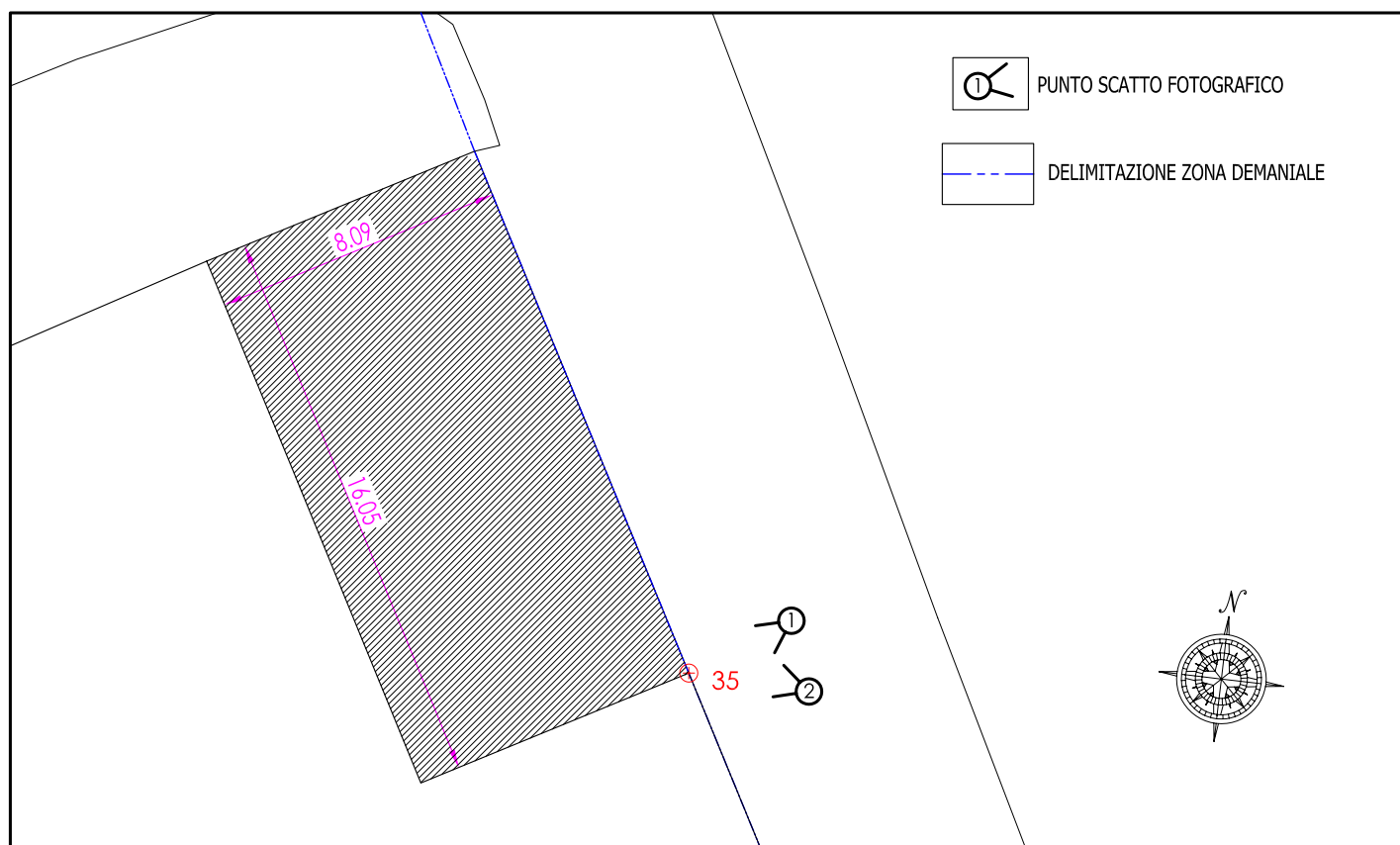
PARTICOLARE MONOGRAFIE
